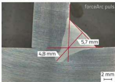
Figure 4 : Caractéristiques de pénétration forceArc puls
