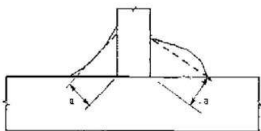
Figure 4.3 - Épaisseur de la soudure en angle
