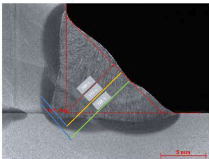
Soudure en angle « normale »
