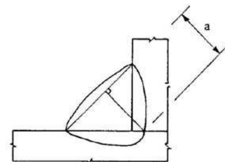
Figure 4.4 – Épaisseur de la soudure en angle avec pénétration profonde
